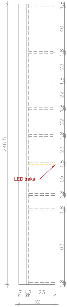
P1 – PRESEK ORMARA
