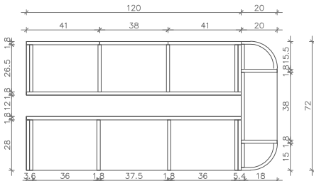
P6&P7 – OSNOVA NAMEŠTAJA U DEČIJOJ SOBI
