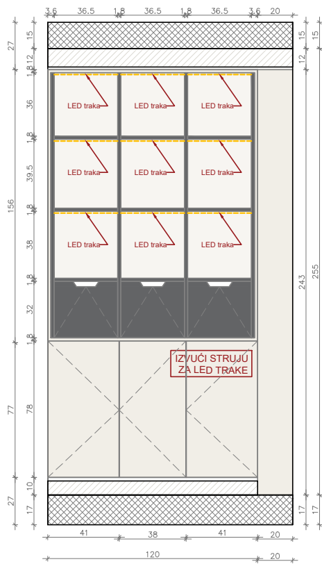
P7 – PRESEK NAMEŠTAJA P7 – IZGLED NAMEŠTAJA U DEČIJOJ SOBI
