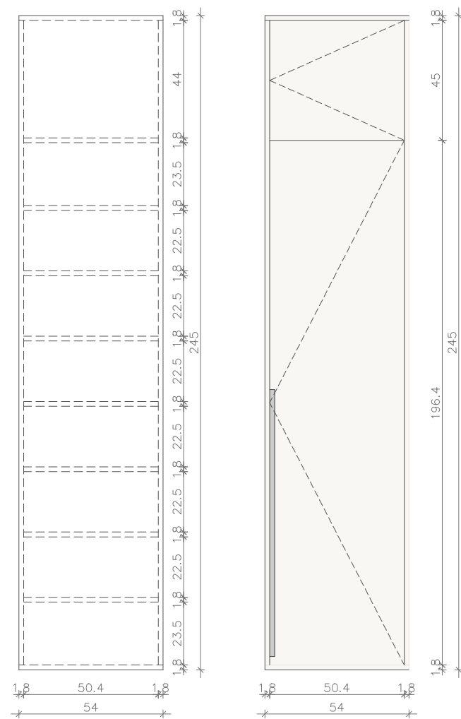
P1 – PRESEK I IZGLED ORMARA
