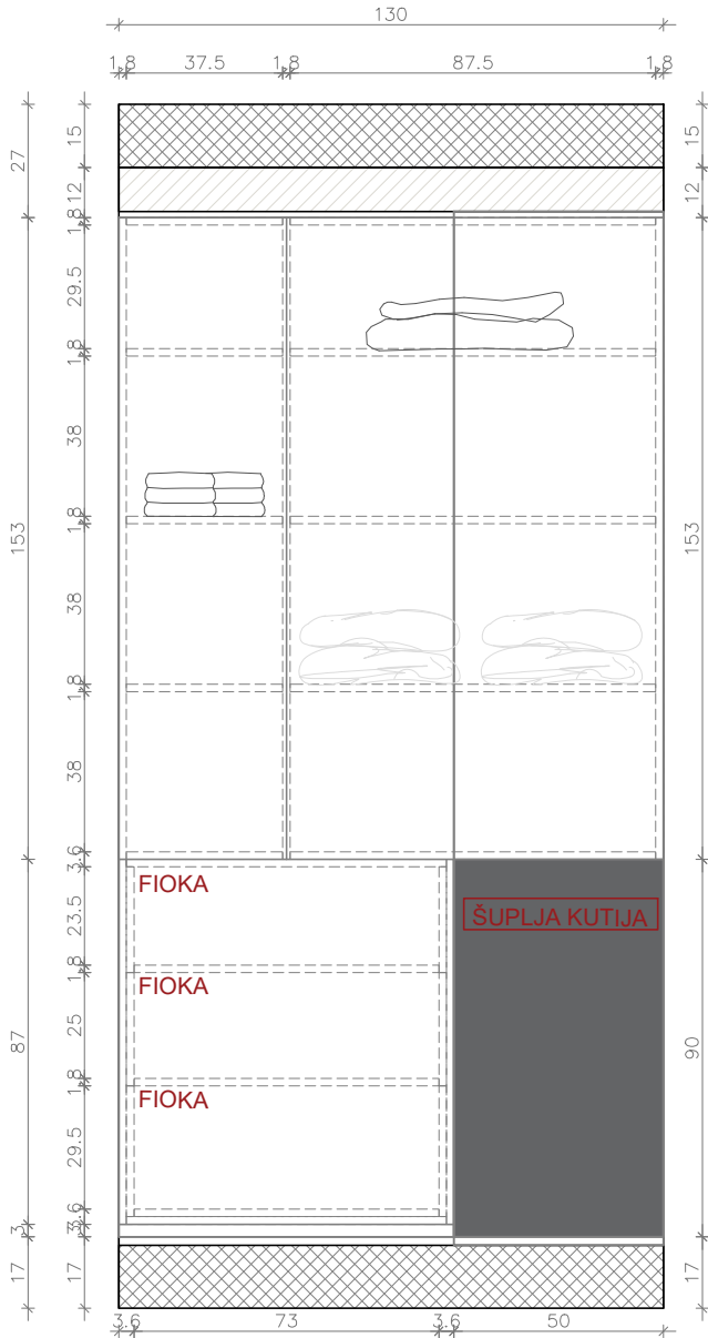
P5 – OSNOVA PLAKARA U DEČIJOJ SOBI
