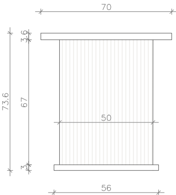
S – IZGLED STOLA
