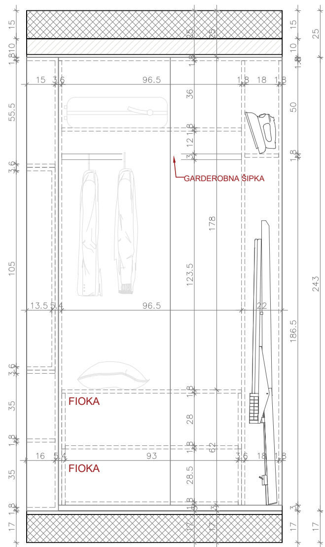
P8 – PRSEK PLAKARA U SPAVAĆOJ SOBI
