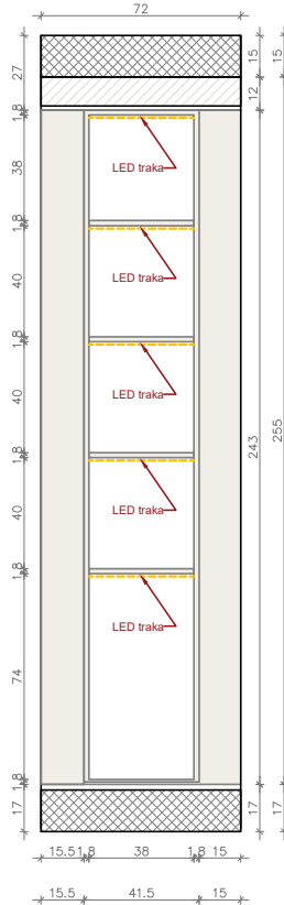
P6 – IZGLED POLICE U DEČIJOJ SOBI
