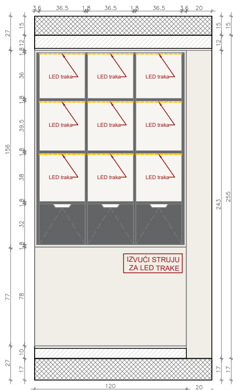
P7 – PRESEK NAMEŠTAJA P7 – IZGLED NAMEŠTAJA U DEČIJOJ SOBI
