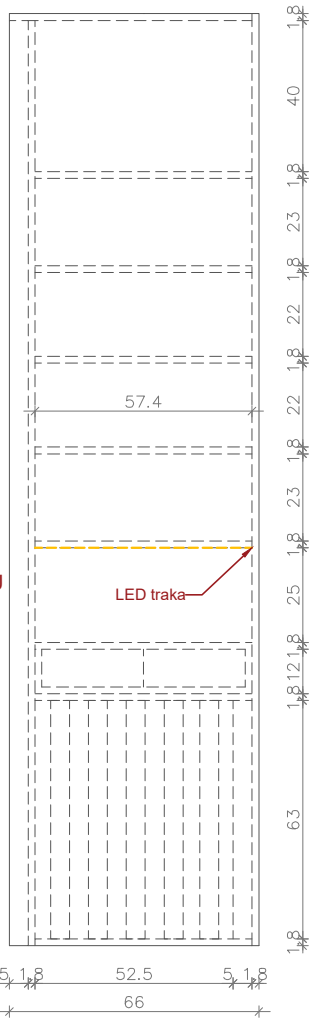
P1 – PRESEK ORMARA
