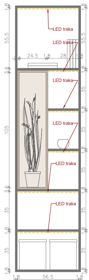
P8 – IZGLED BOČNE POLICE
