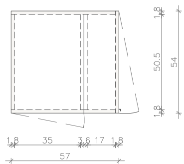
P1 – OSNOVA ORMARA
