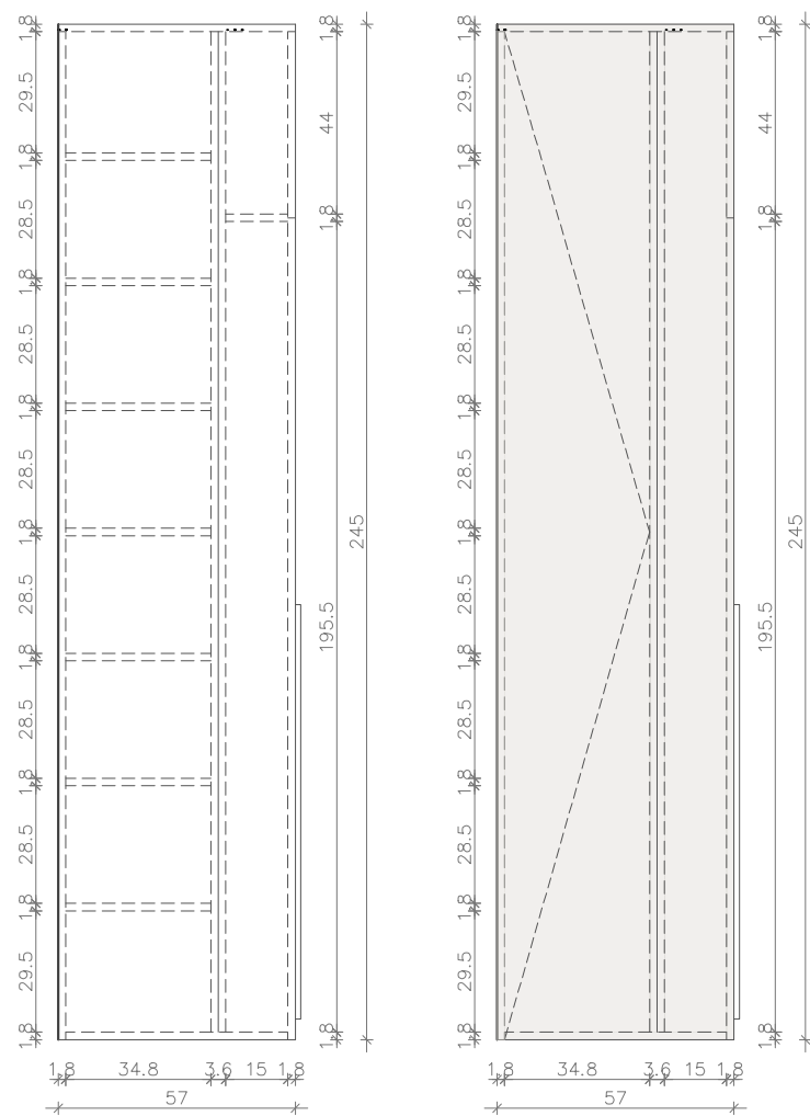
P1 – PRESEK I IZGLED ORMARA
