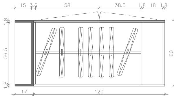
P8 – ONOVA PLAKARA U SPAVAĆOJ SOBI
