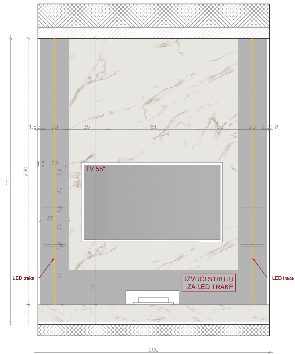
TV – IZGLED TV ZIDA
