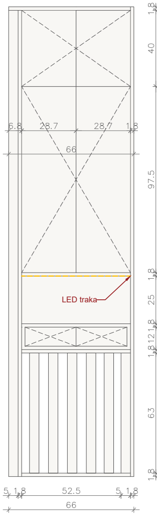
P1 – IZGLED ORMARA
