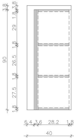
K – IZGLED ŠANK
