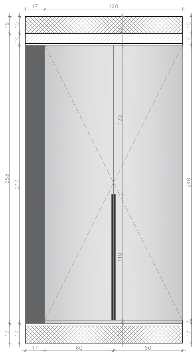
P8 – IZGLED PLAKARA U SPAVAĆOJ SOBI
