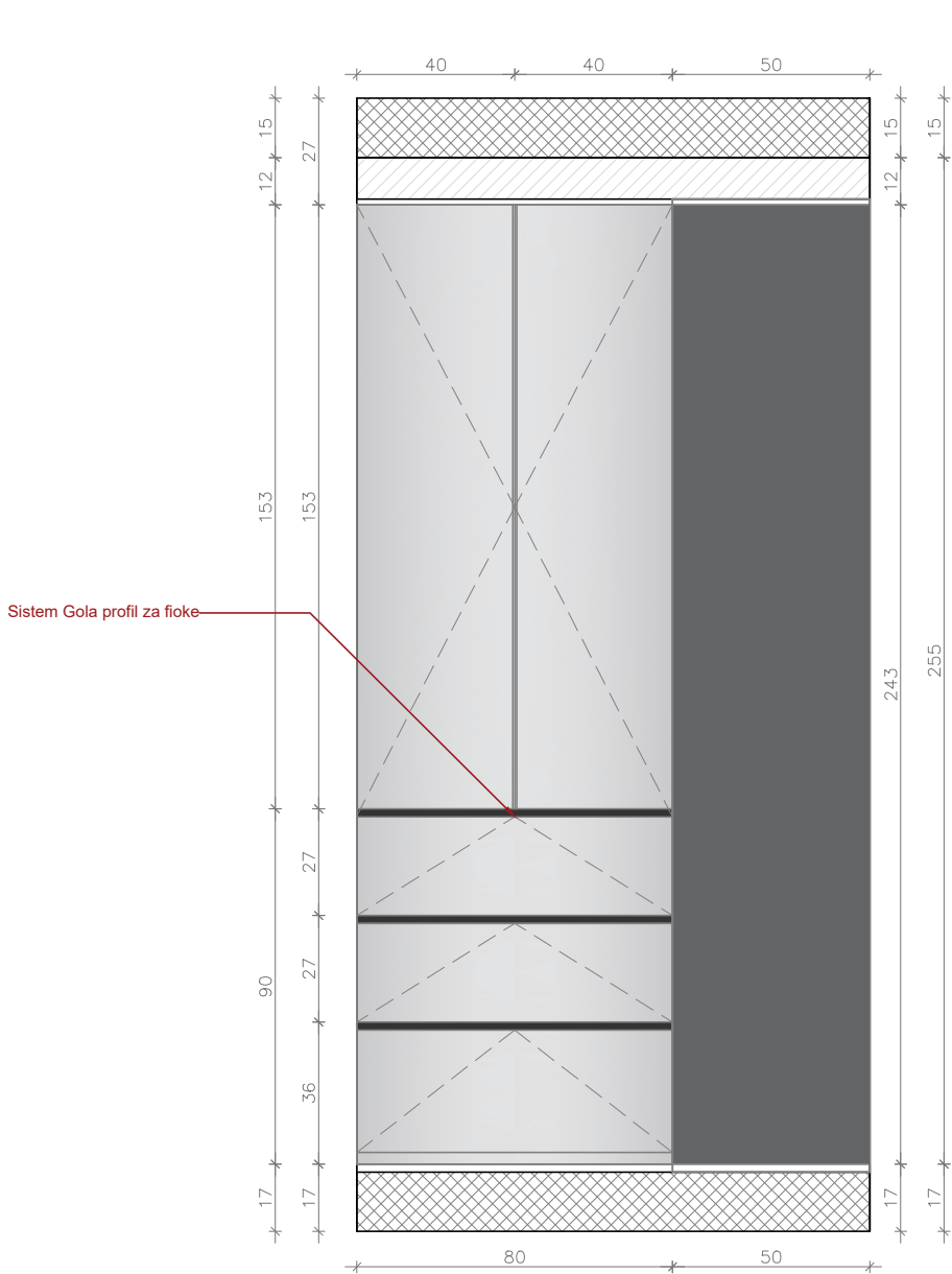
P5 – IZGLED PLAKARA U DEČIJOJ SOBI
