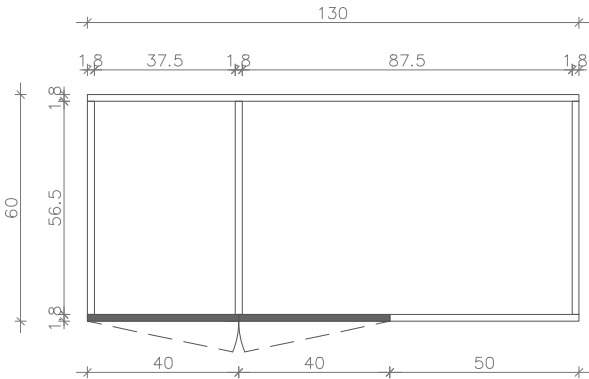
P5 – OSNOVA PLAKARA U DEČIJOJ SOBI
