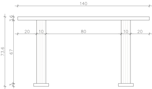
S – IZGLED STOLA
